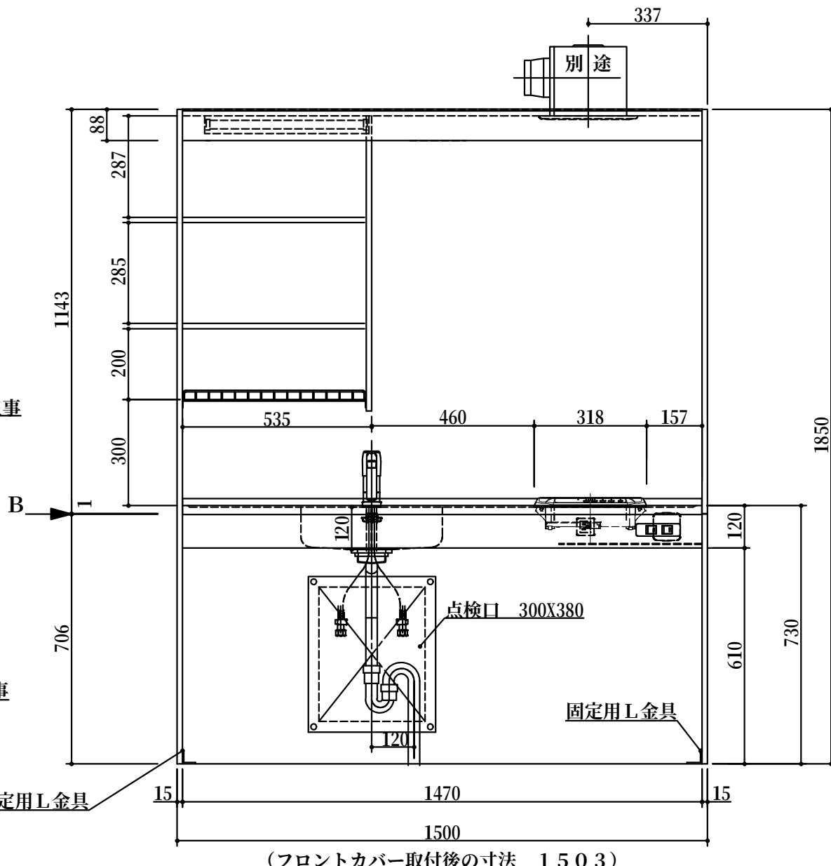
(フロントカバー取付後の寸法 1503)
