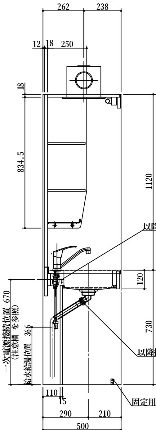
(フロントカバー取付後の寸法 502)
